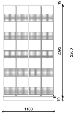
00.16.01 Apothekerschrank Innenaufteilung
