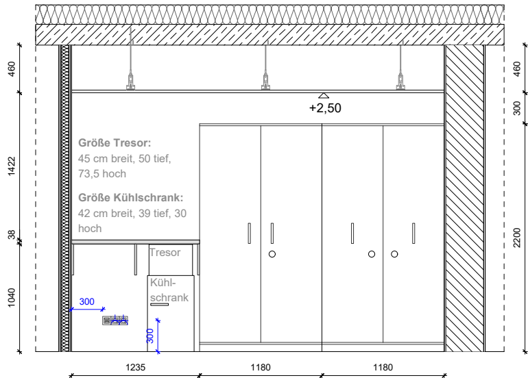
Ansicht medizinisches Lager: 1,18er Schränke + Board
