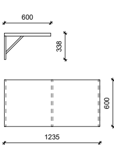
00.16.03 Ablageboard
