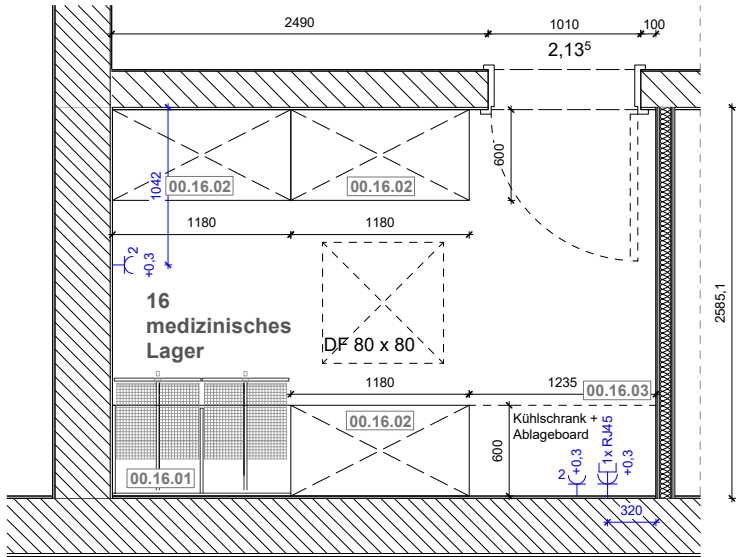
Grundriss medizinisches Lager: 1,18er Schränke, Anschlag Tür 10 cm, TB-Wand um 10 cm Richtung Desinfektion verschoben
