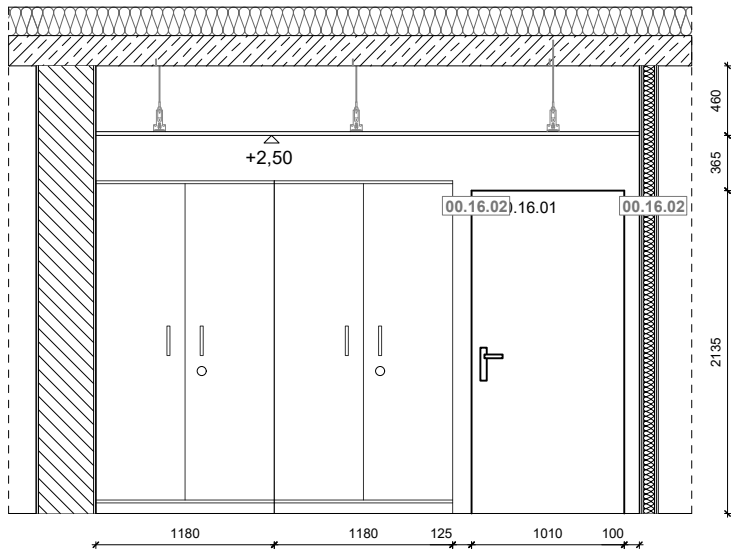
Ansicht medizinisches Lager: 1,18er Schränke
