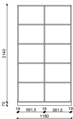
00.16.02 Medizinschrank Innenaufteilung
